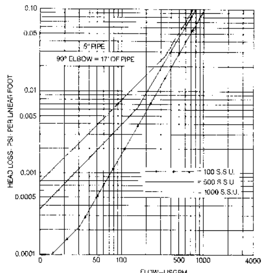
5" PIPE
